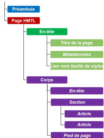
Structure logique globale d'un fichier HTML (les éléments en italique sont facultatifs)
