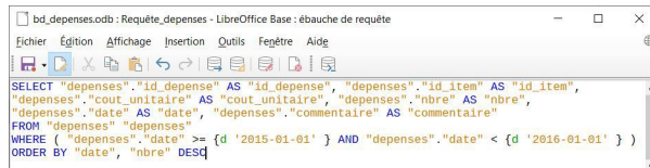
Requête SQL dans Base
