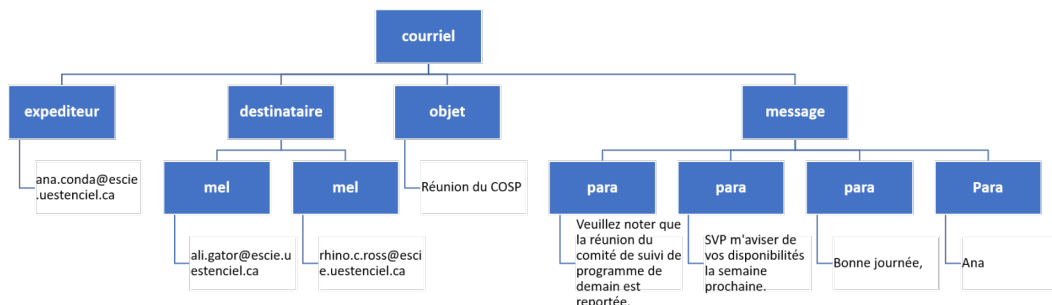
Structure logique d'un courriel
